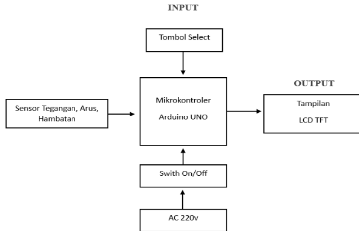
Gambar 5 Blok Diagram Alat
