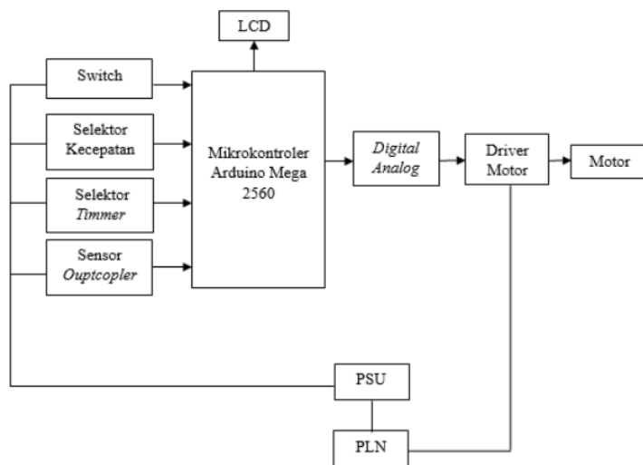
Gambar 2. Blok Diagram Alat
